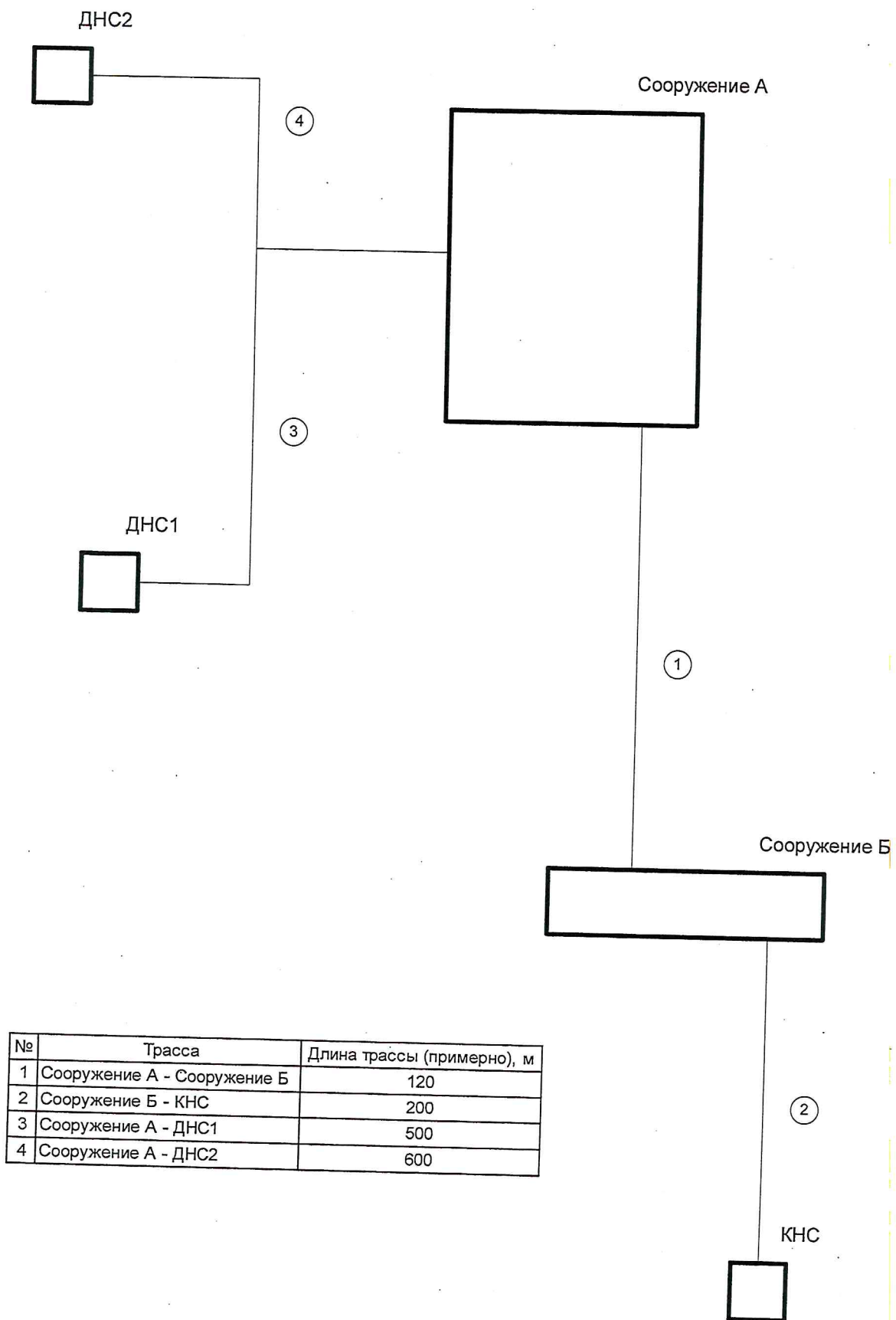
Рис. 1. Расположение диспетчеризируемых объектов
